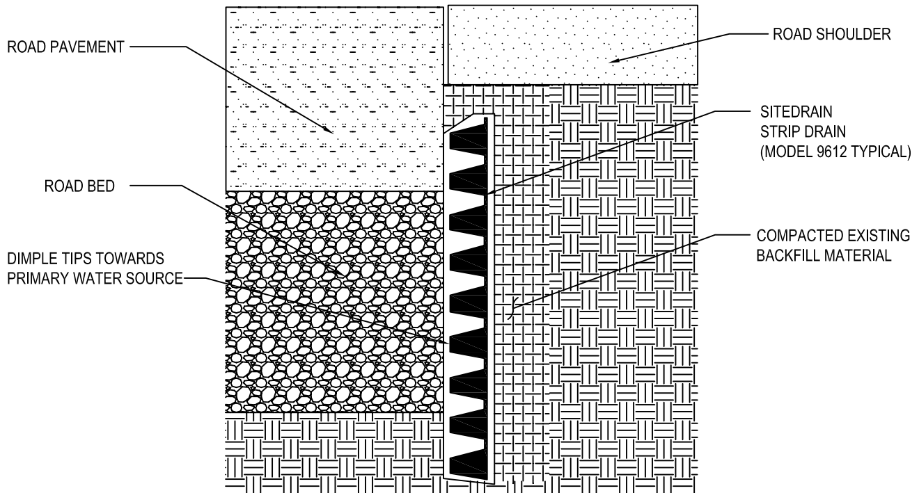
ROADWAY EDGE DRAIN
